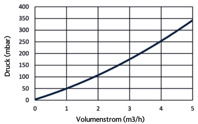
Savo 15 SG-M Druckverlustkurve
