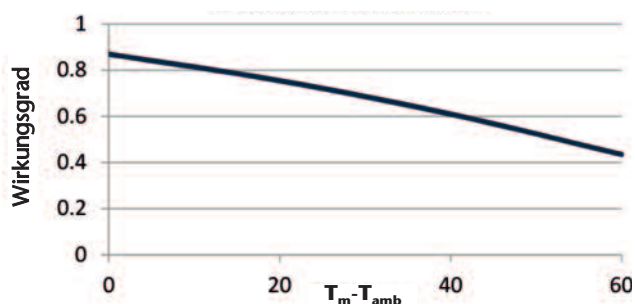
Wirkungsgrad je Temperaturdifferenz: Savo 15 SG-M
